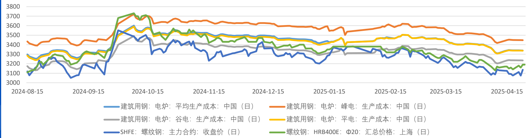
螺纹钢价格vs电炉成本
