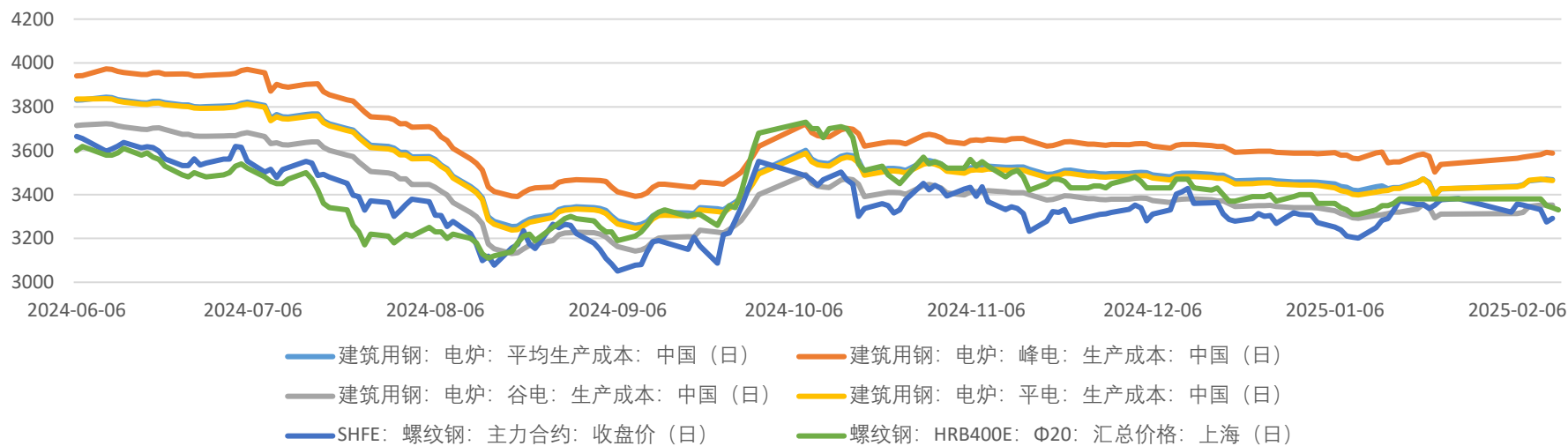
螺纹钢价格vs电炉成本
