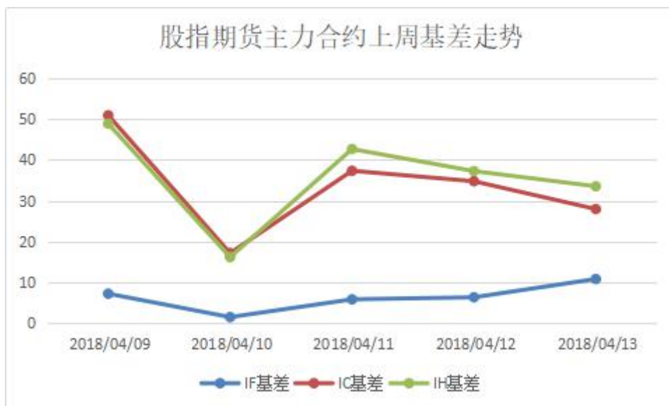
图 2：IF、IC、IH 合约基差走势
