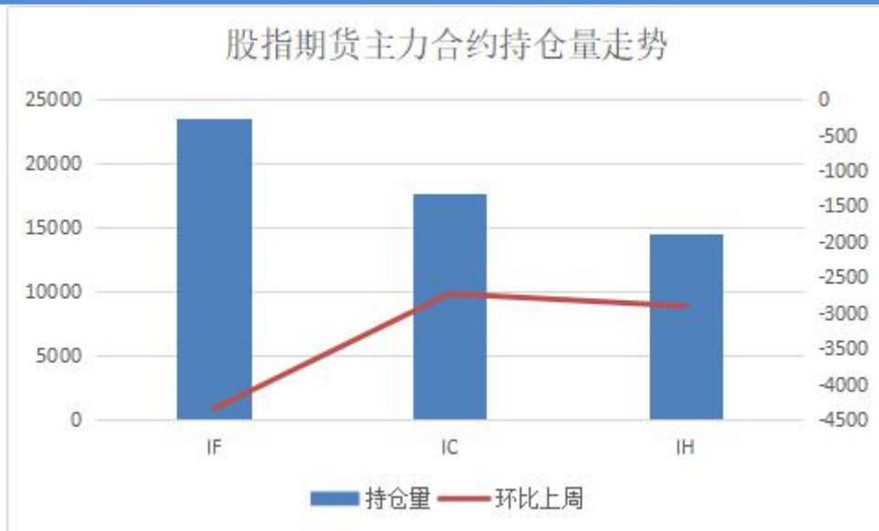
图 3：IF、IC、IH 主力合约上周仓位变化
